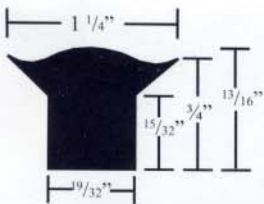
R221 RUBBER, EPDM 275-300- Temp. Deg. F
