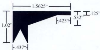
R241 EPDM RUBBER 275-300 - Temp. Deg. F
