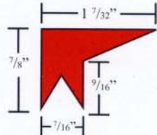
S212 SILICONE 350-450 - Temp. Deg. F
