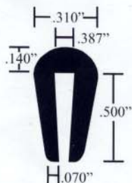
R240 EPDM RUBBER 275-300 - Temp. Deg. F
