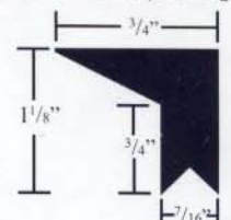
R230 EPDM RUBBER 275-300 - Temp. Deg. F
